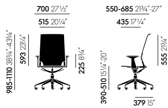
Meda Chair, met armleuningen
