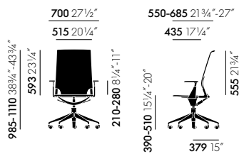
Meda Chair, met in de hoogte verstelbare armleuningen
